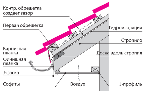
Подшивка свеса
