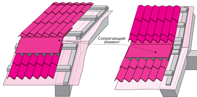
Устройство изломов кровли
